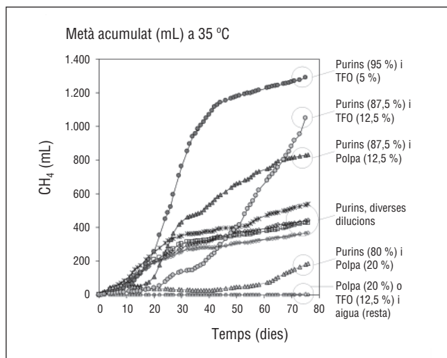
FIGURA 2. Produccions mitjanes de \text{CH}_4 de la codigestió en discontinu de diferents proporcions de purins de porc amb terres filtrants d'oli d'oliva (TFO) o amb polpa de pera
